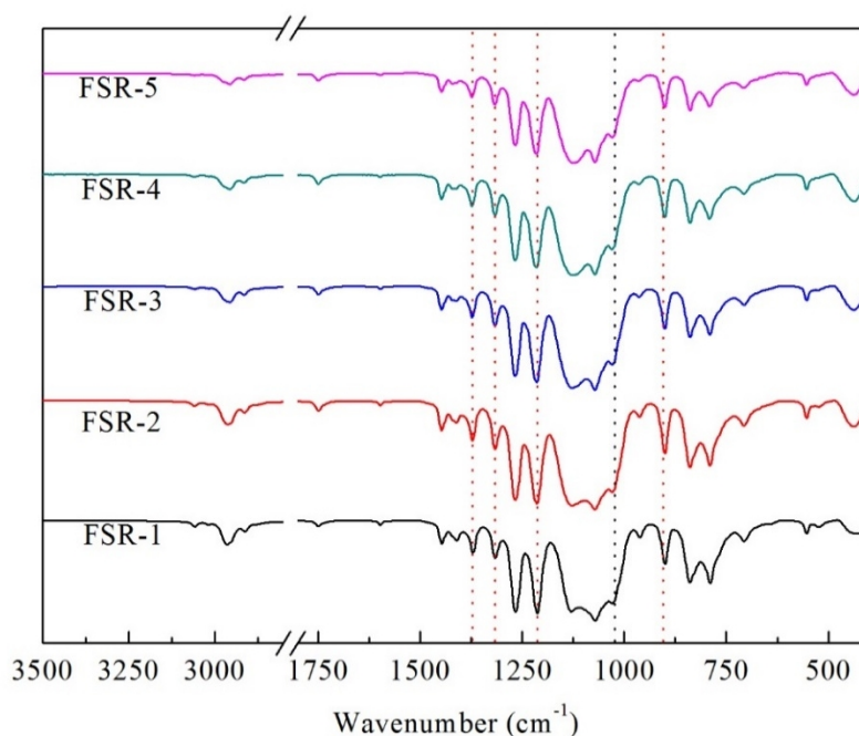
Fig.1. FTIR spectra of FSR
